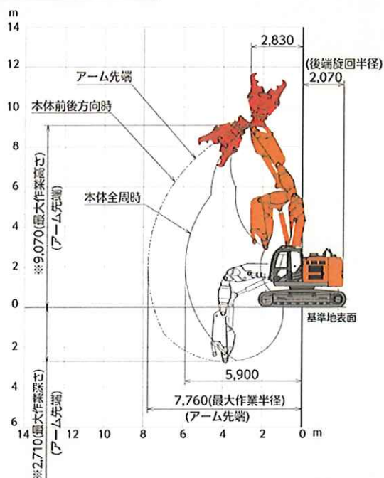
3 段ショートリーチ
