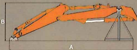
ツーピースブーム
