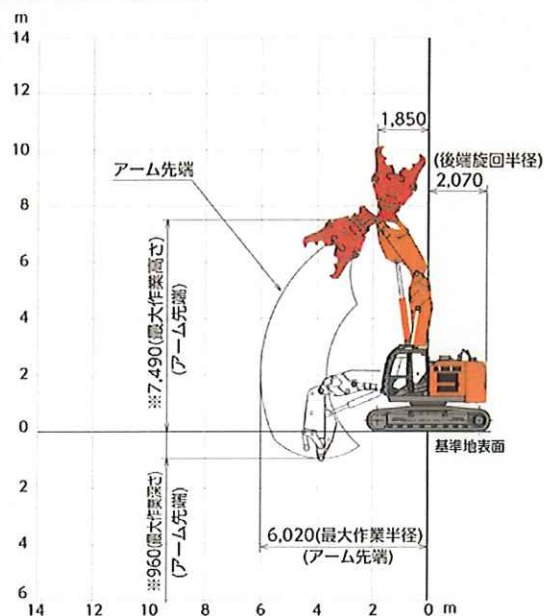
2 段ショートリーチ
