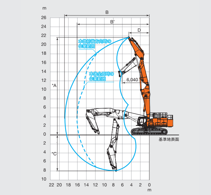
ツーピースブームフロント仕様
