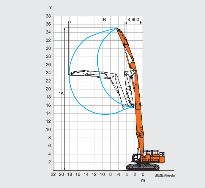
モンスタハイリフトフロント仕様 (35 m 仕様)
