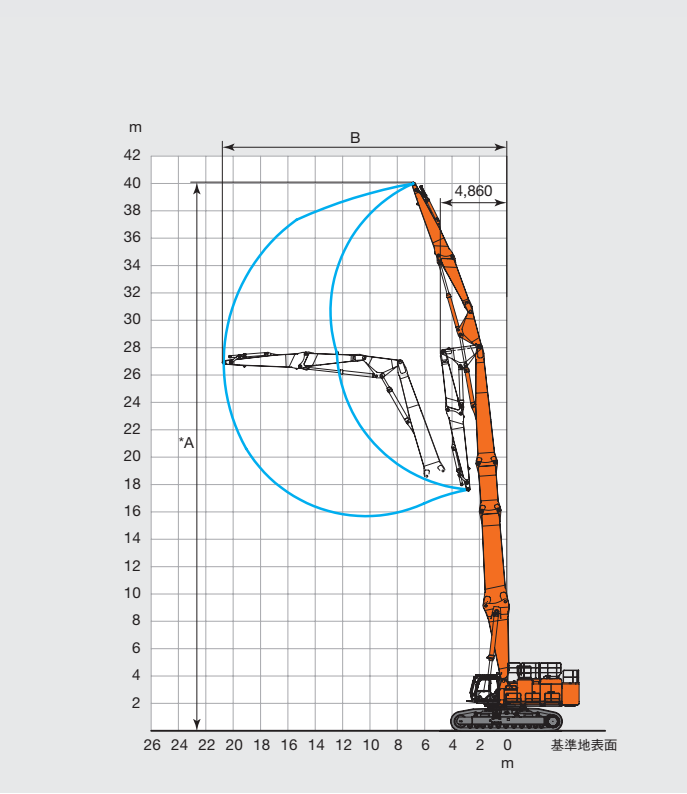
モンスタハイリフトフロント仕様 (40 m 仕様)
