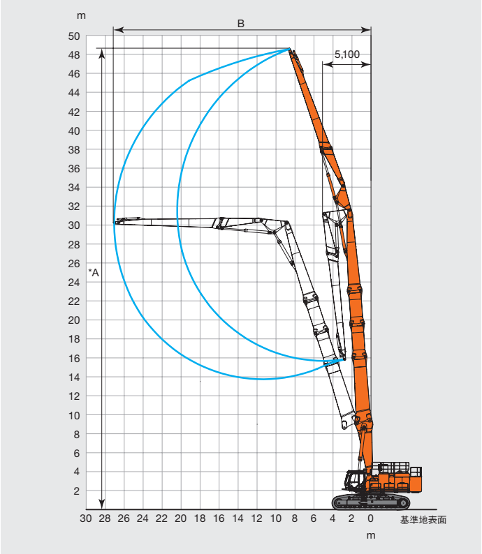
ハイリフトフロント仕様 (48.5 m 仕様)
