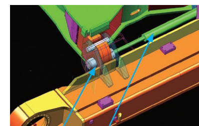
ピン伸縮用シリンダ サイドフレーム締結ピン
