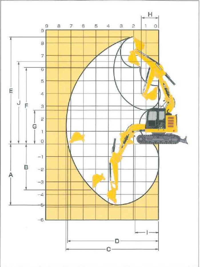
作業範囲 (単位: mm)
