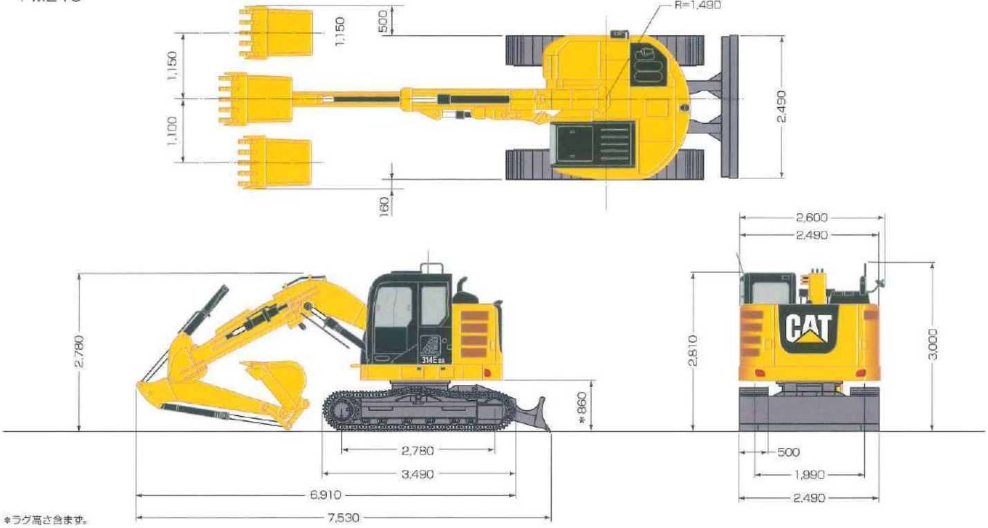
外形図 (単位: mm)
